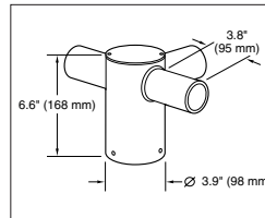
PT-3 (90) 90° Triple
