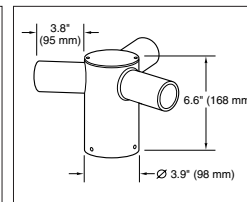
PT-3 (120) 120° Triple
