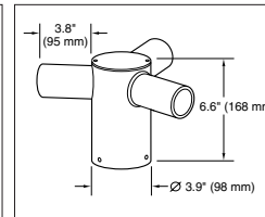
PT-3 (120) 120° Triple
