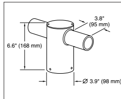
PT-2 (180) 180° Twin
