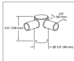
PT-2 (90) 90° Twin
