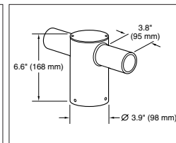
PT-2 (180) 180° Twin
