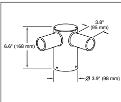
PT-2 (90) 90° Twin
