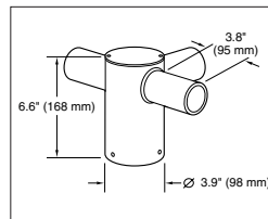
PT-3 (90) 90° Triple
